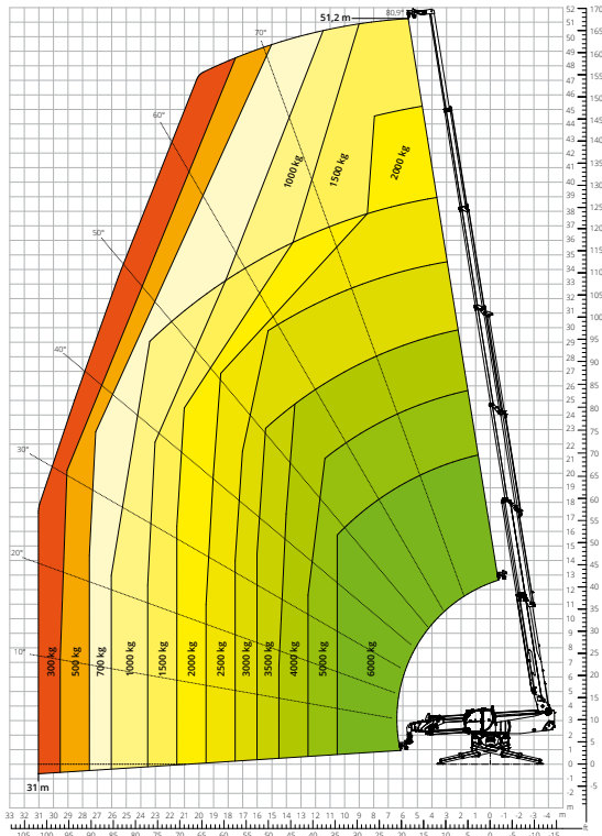
Abaque de charge avec CROCHET 6 000 kg ATT - 05 - 001
