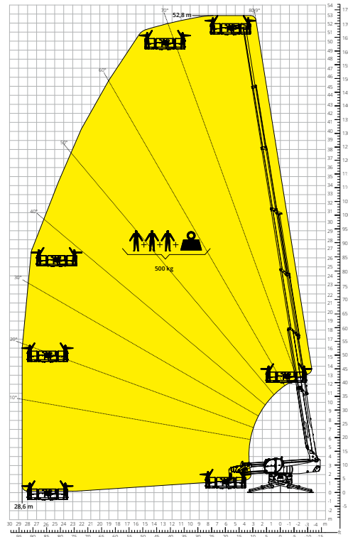
Abaque de charge avec PANIER NACELLE EXTENSIBLE ROTATIF 500 kg ATT-01-007
